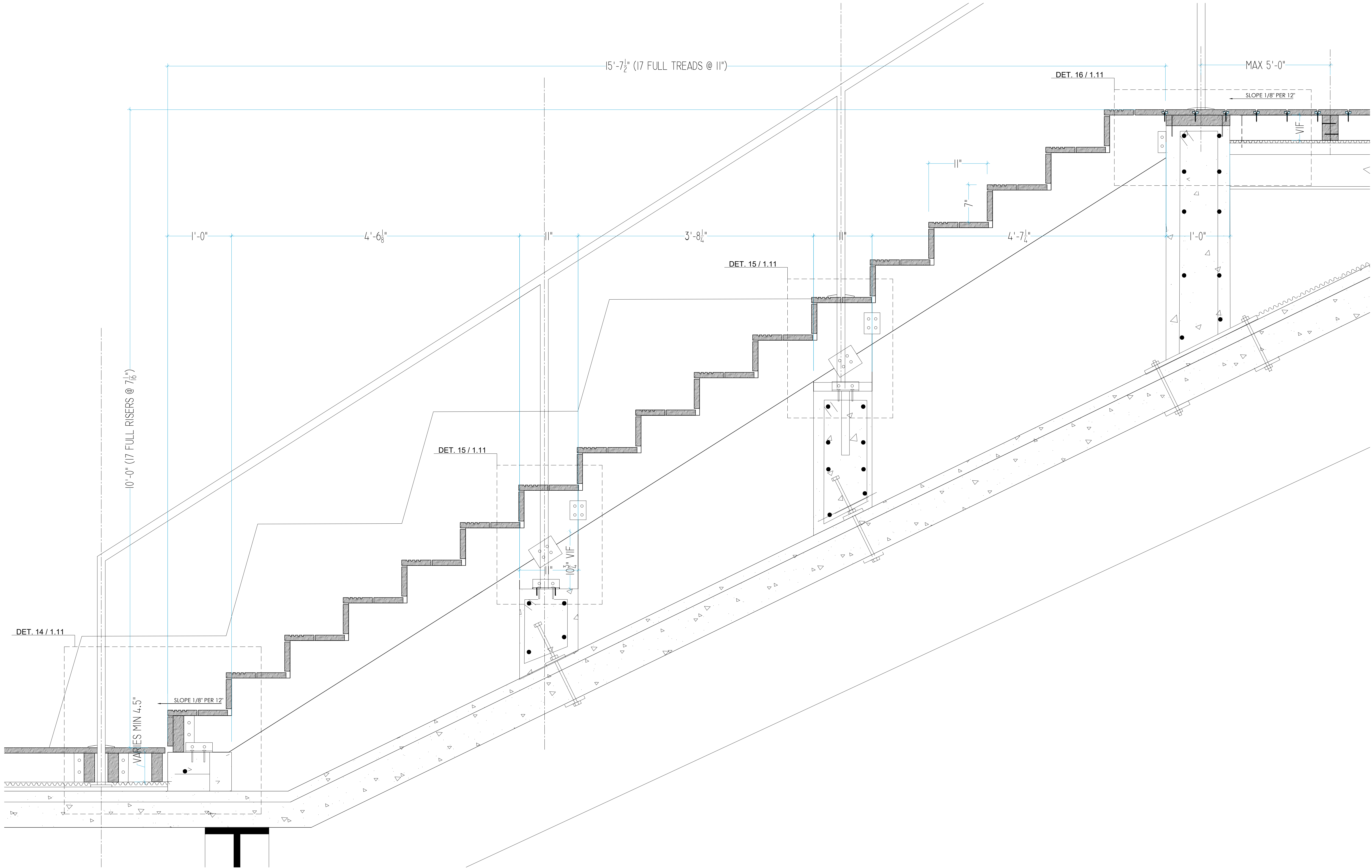
WOOD STAIRS - SECTION A-A Scale: 1-1/2" = 1' - 0"
